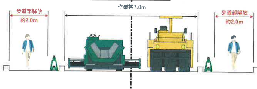
車道部作業形態図
